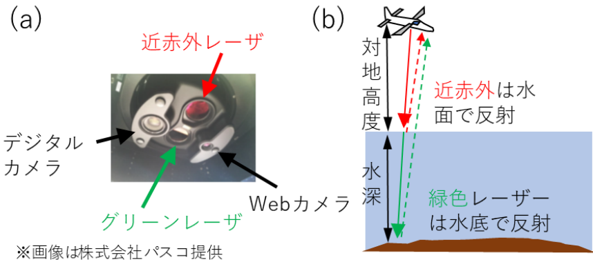
図. (a) 航空レーザー測深 (ALB) のセンサーと (b) 計測の仕組み
