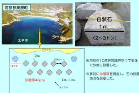
図1 単体礁に用いた石材と配置
