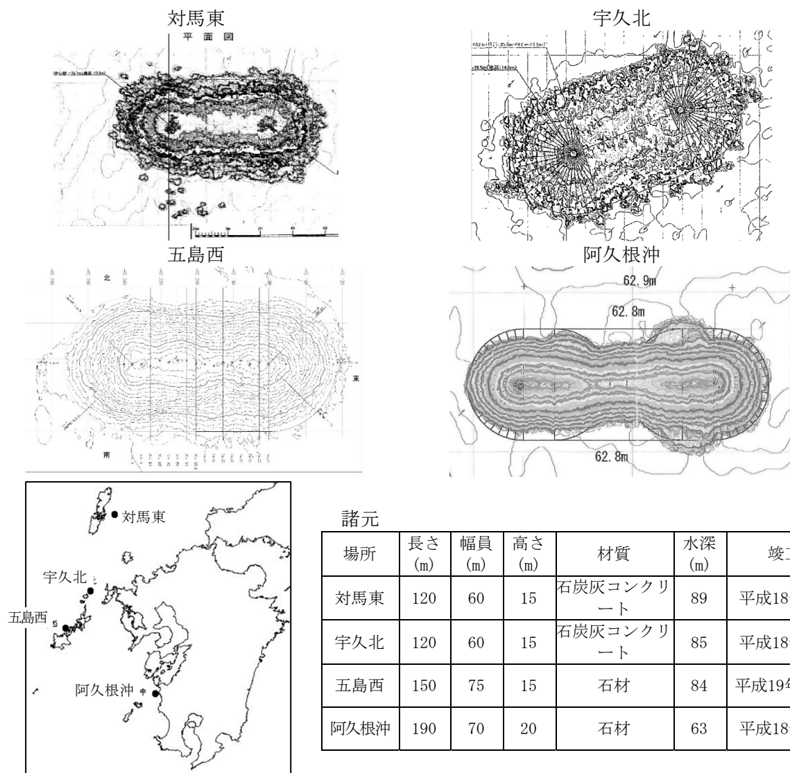
図 5-6 マウンド礁の概要
