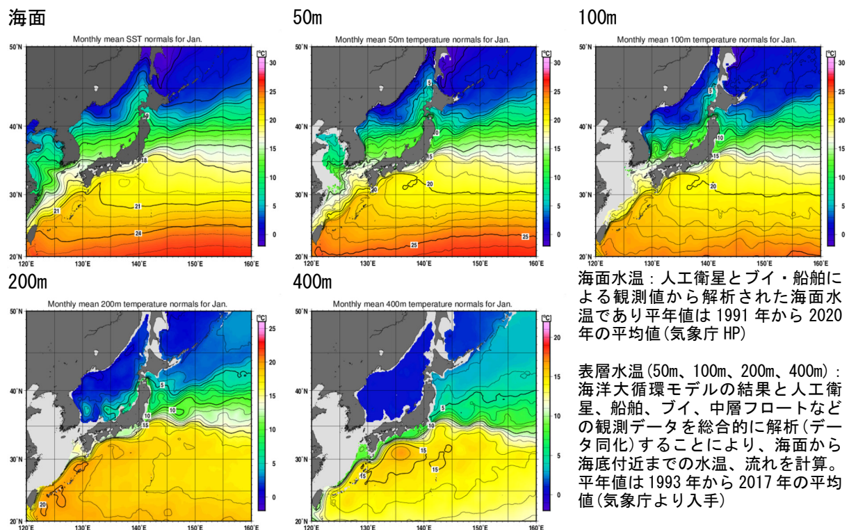
図 5.2 現況水温に用いた日本近海の平年値の例
