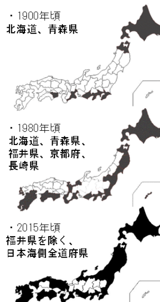
■ 藻場衰退域を抱える都道府県 水産庁;改訂磯焼け対策ガイドライン(2015)より 図 3.9 藻場衰退域を抱える都道府県の推移
