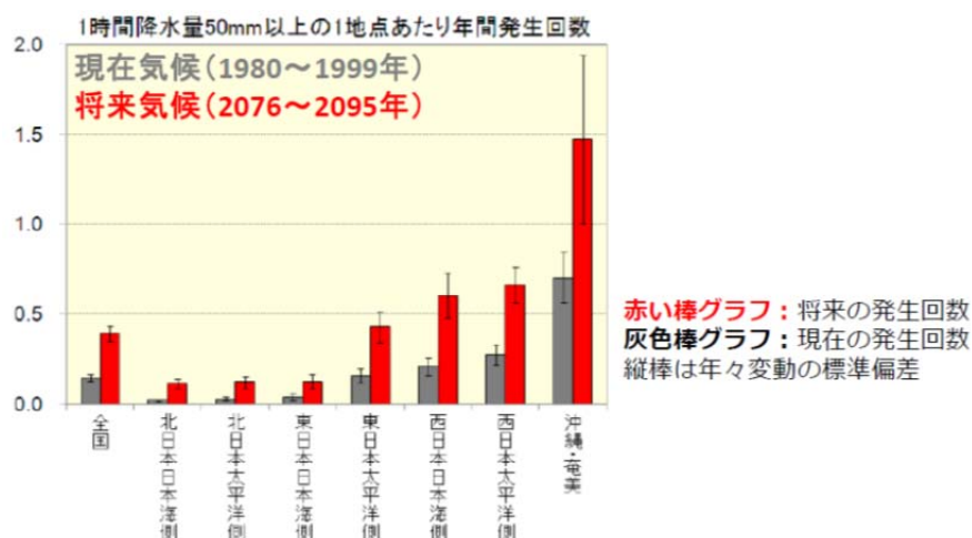
図 2.7 地域別の短時間強雨の発生頻度の変化
