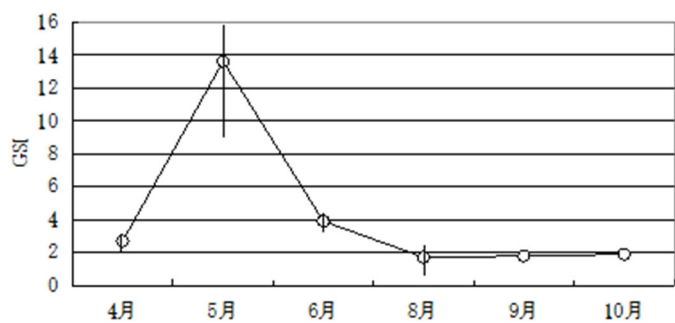
図 5-7 ウマヅラハギの GSI の季節変化
