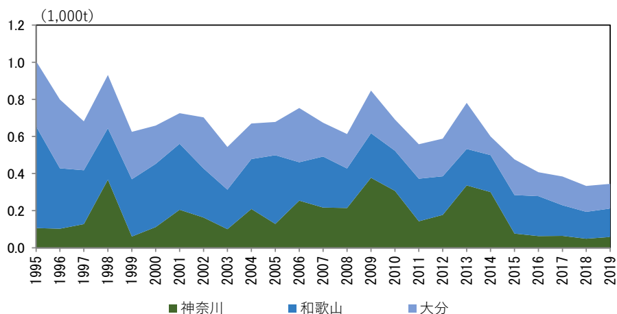
図 5-24 資源評価実施県のイサキの漁獲量の推移
