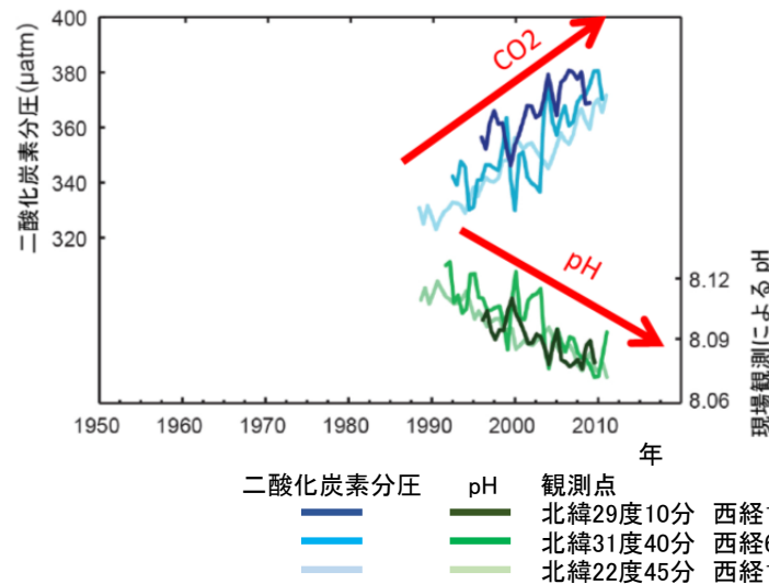
図 2.3 海面の二酸化炭素と pH 9
