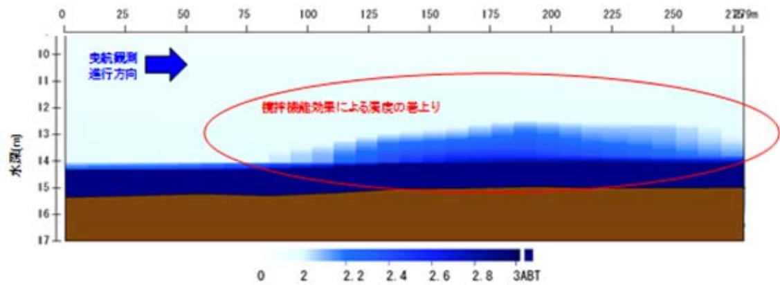
図4 濁りの巻上げの状況
