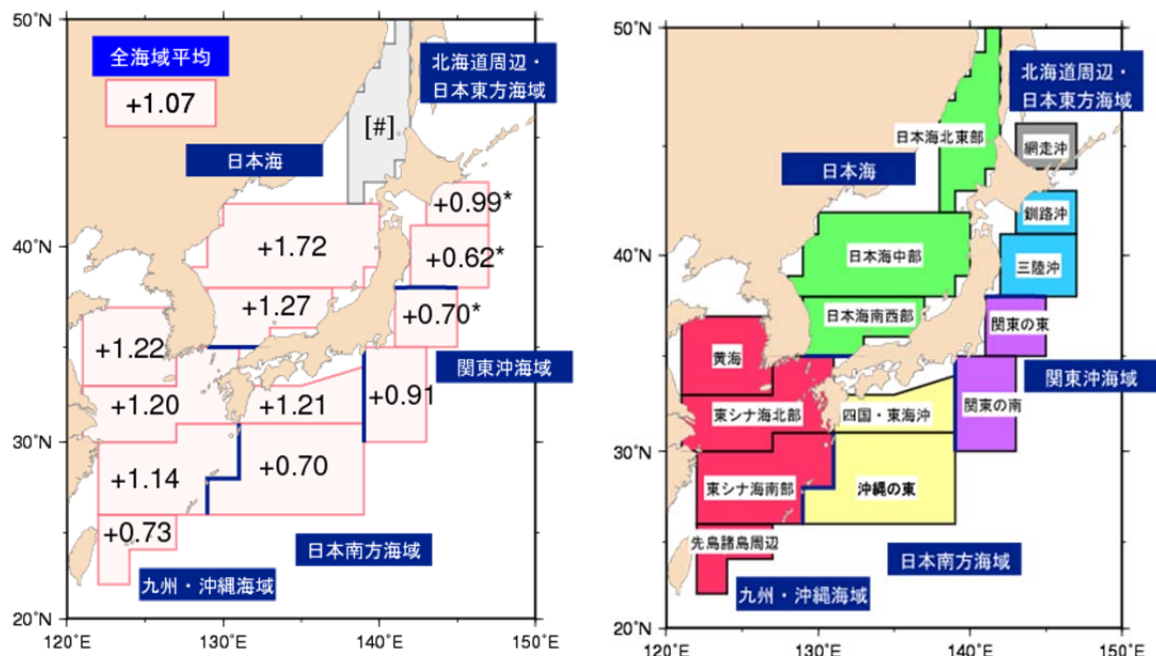
図 2.1 日本近海の平均海面水温（年平均）の長期変化傾向（ ^{\circ}\text{C}/100 年）（左図）と海域区分（右図）
