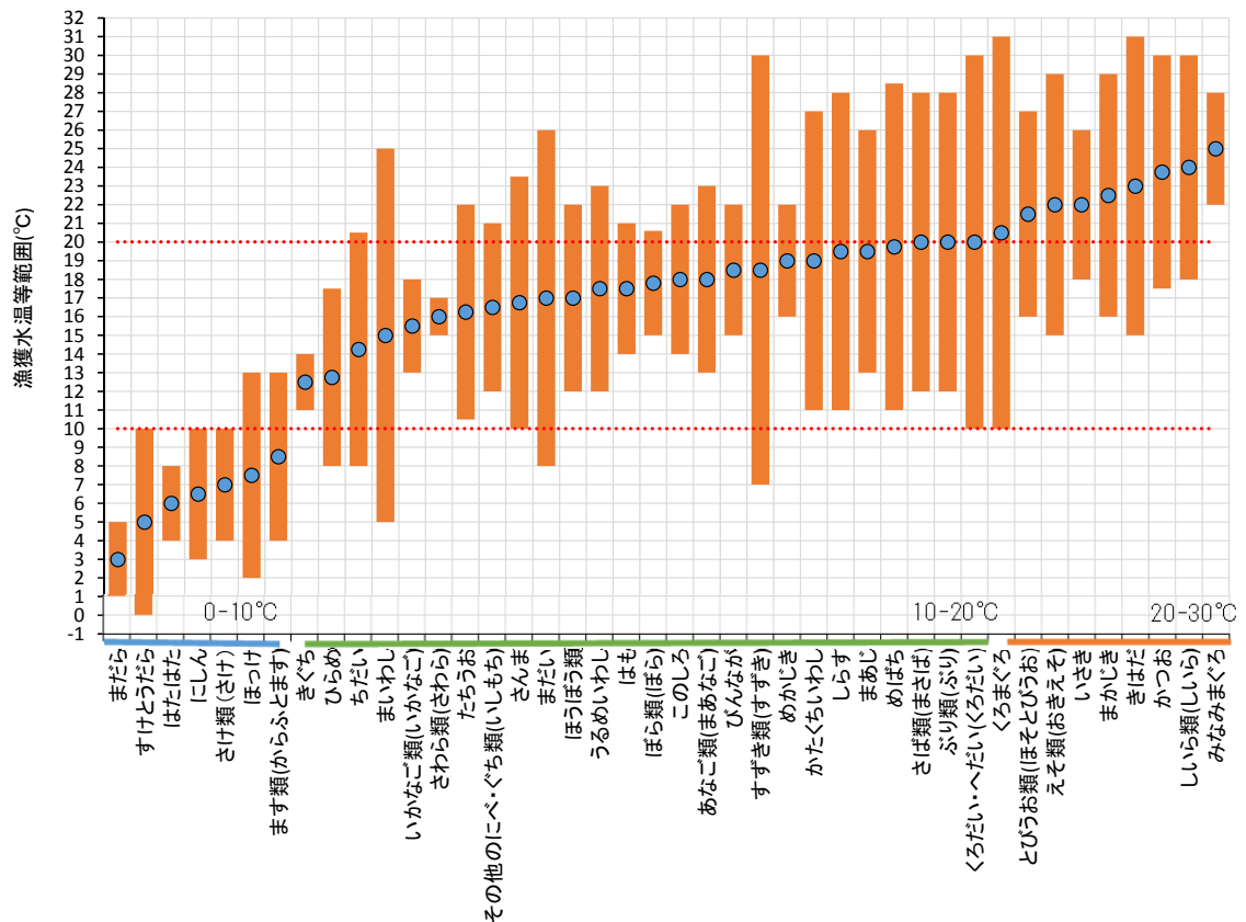
図 3. 21 魚類の漁獲水温等の範囲
