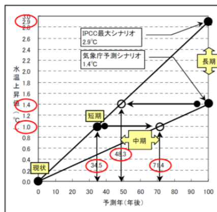
図 3.12 水温上昇のシナリオ
