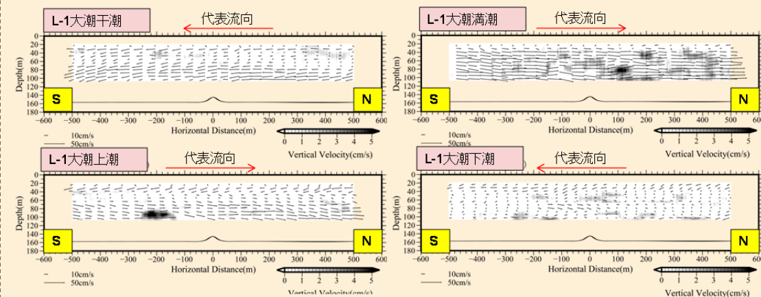
図2 流況の観測結果
