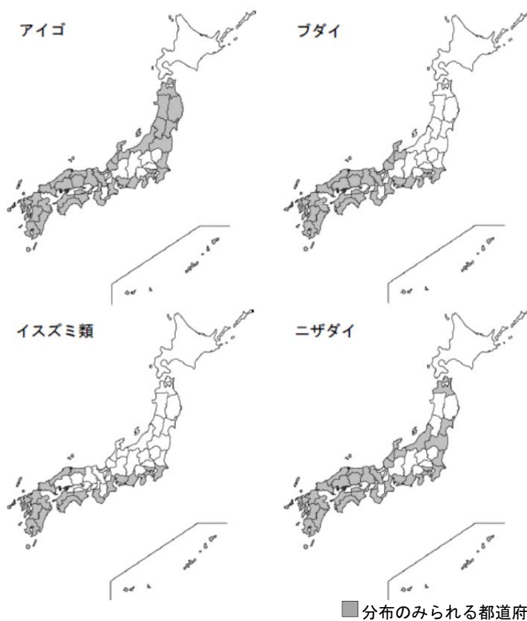
図 3.3 植食性魚類の分布
