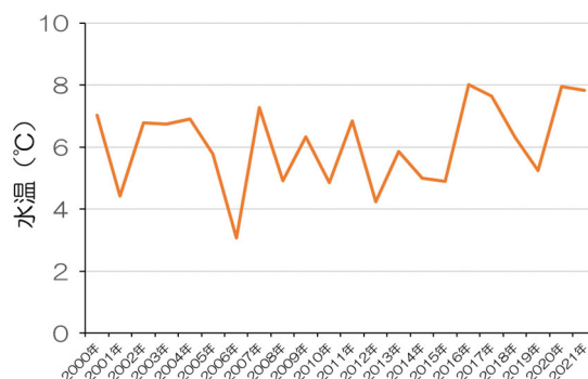
図 5-17 岩手県山田湾の 3 月の平均水温
