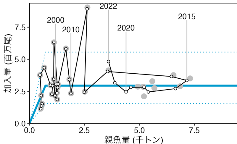
図6 再生産関係
