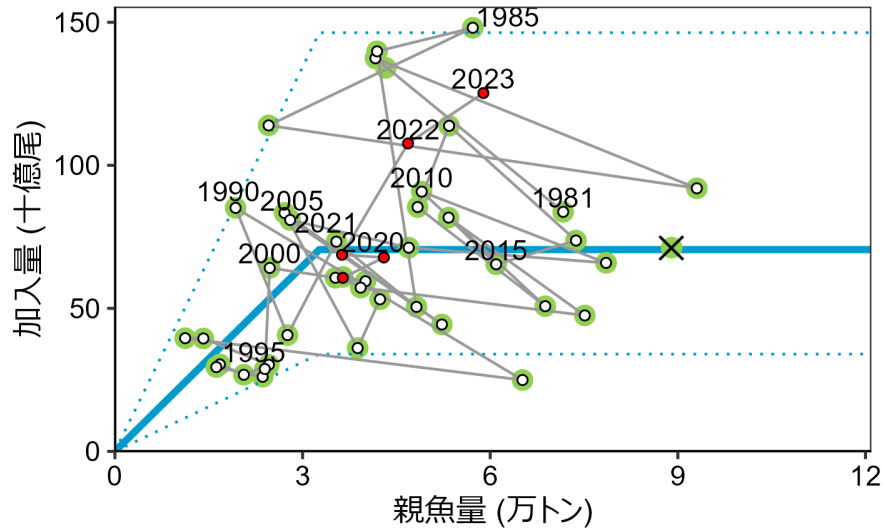
図6 再生産関係
