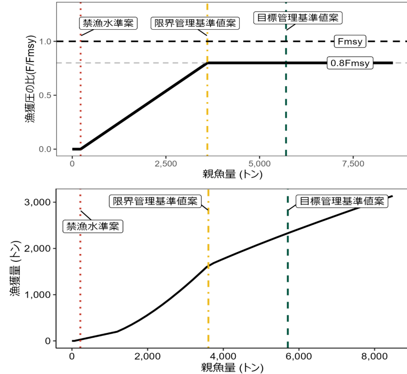
図9 漁獲管理規則案 (上図：縦軸は漁獲圧、下図：縦軸は漁獲量)
