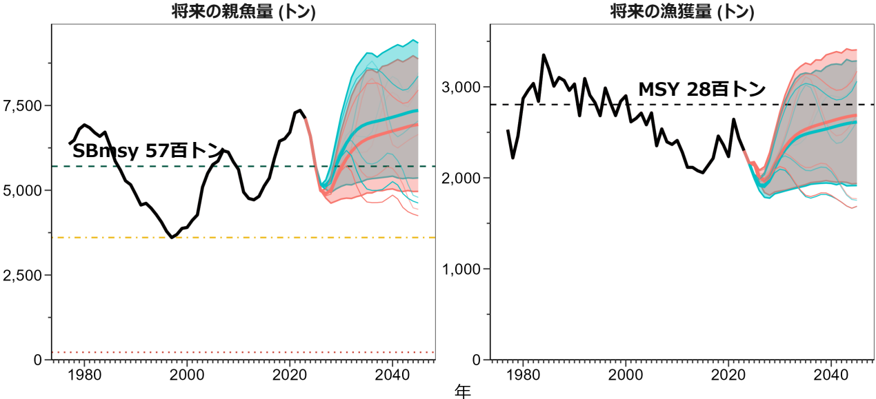
図11 種苗放流を想定した場合の漁獲管理規則案の下での親魚量と漁獲量の将来予測 (現状の漁獲圧は参考)
