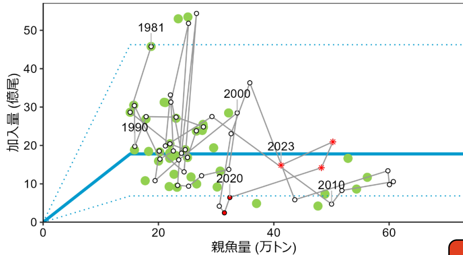
図7 再生産関係
