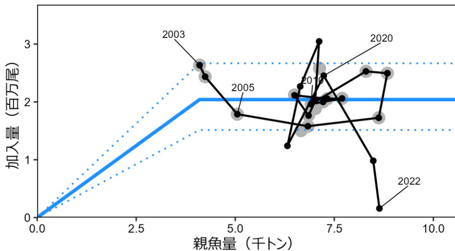
図6 再生産関係
