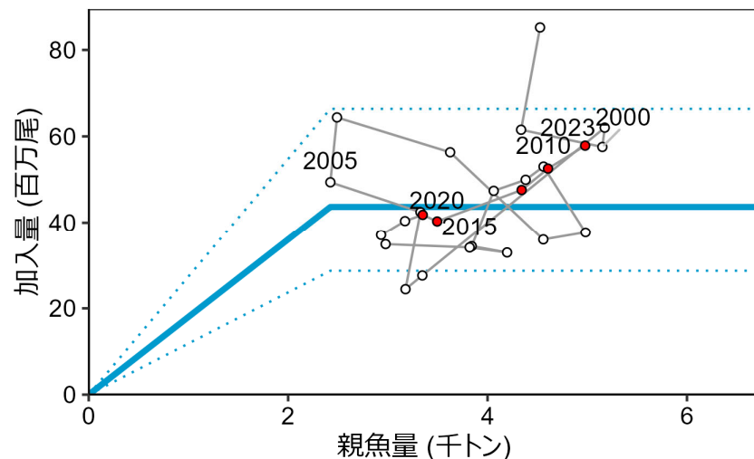
図6 再生産関係
